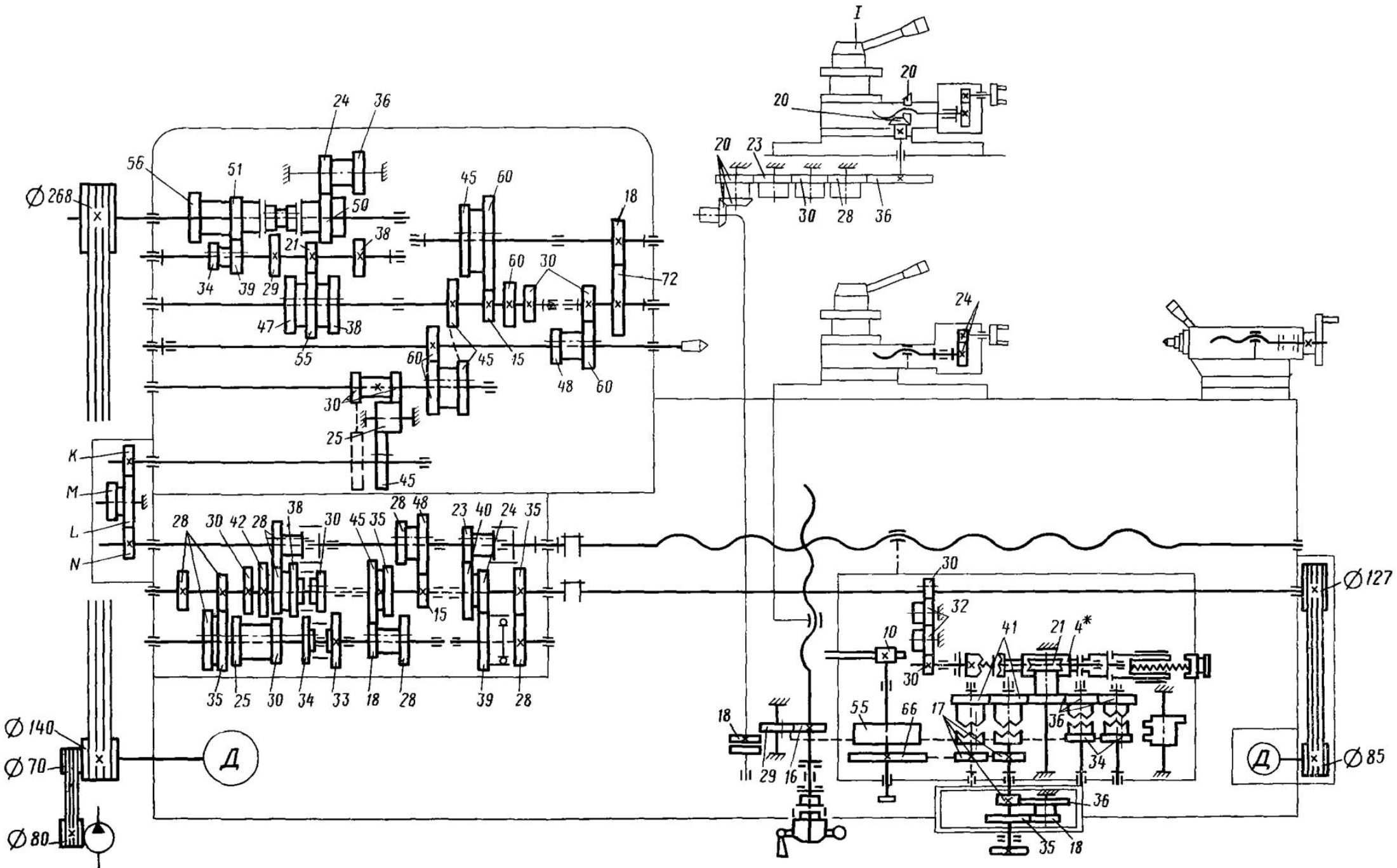
Рис. 40. Кинематическая схема
