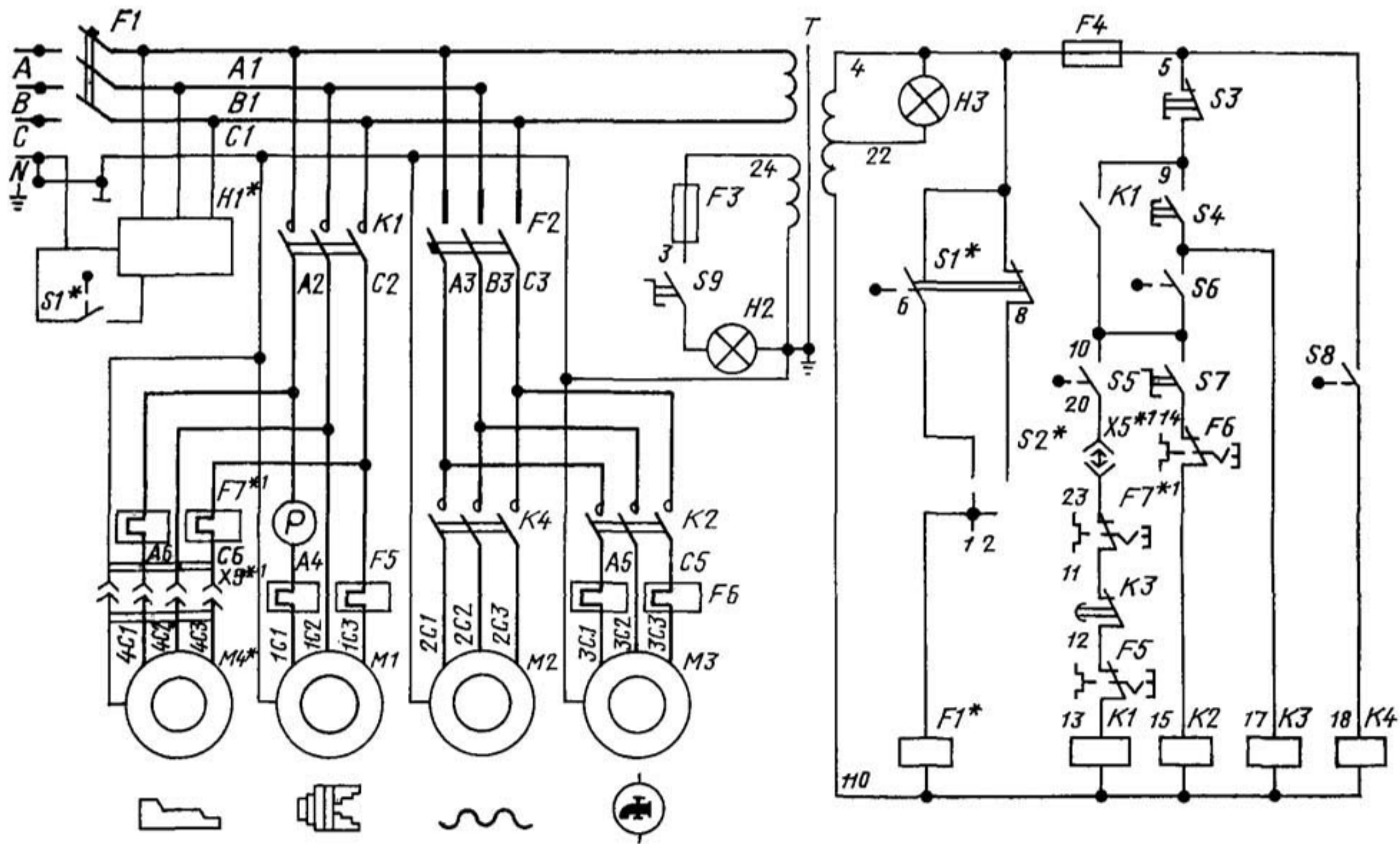
Рис. 4. Схема электрическая принципиальная
